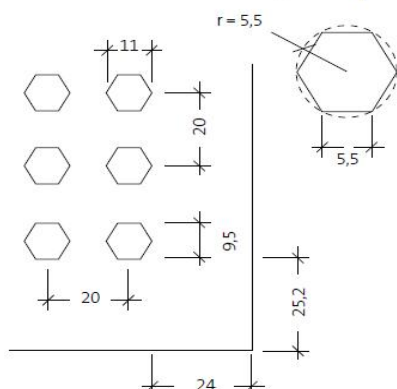
Rozmieszczenie i wielkość perforacji
